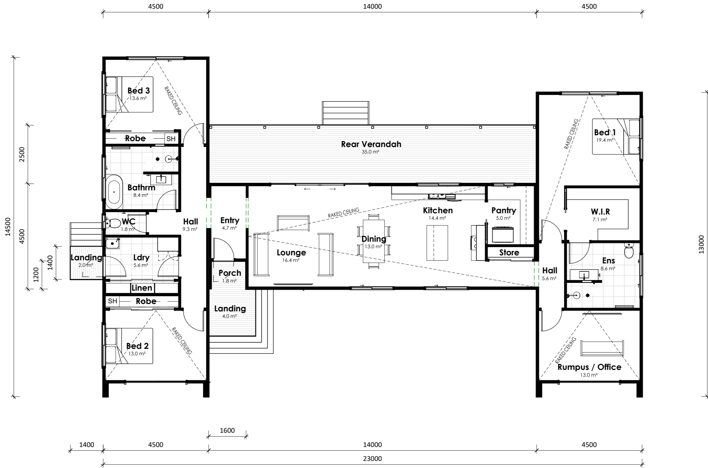
FLOOR PLAN 1 : 100
