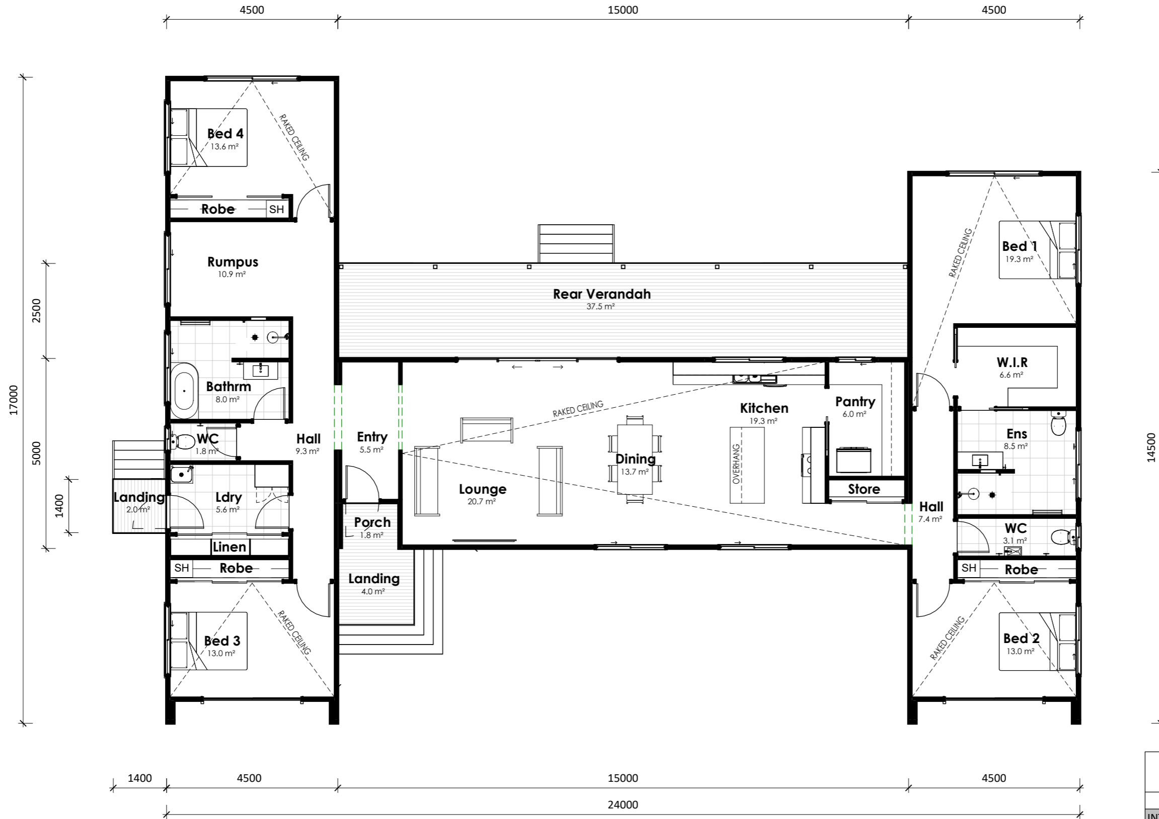
FLOOR PLAN 1 : 100
