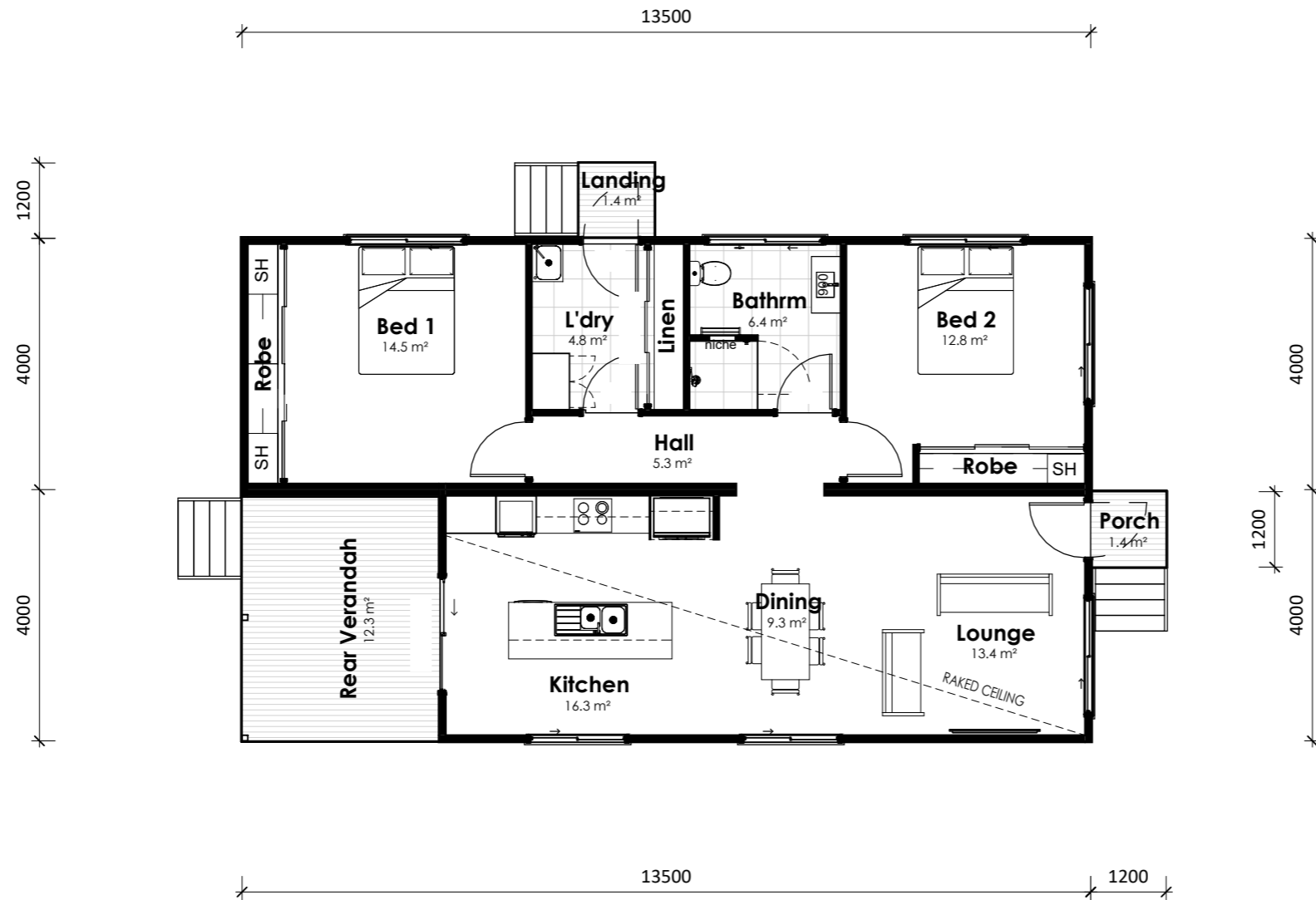
FLOOR PLAN 1 : 100
